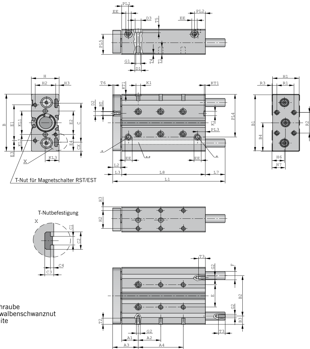
Maßtable (mm) – Baureihe FZK(G) 6020 bis 6032
