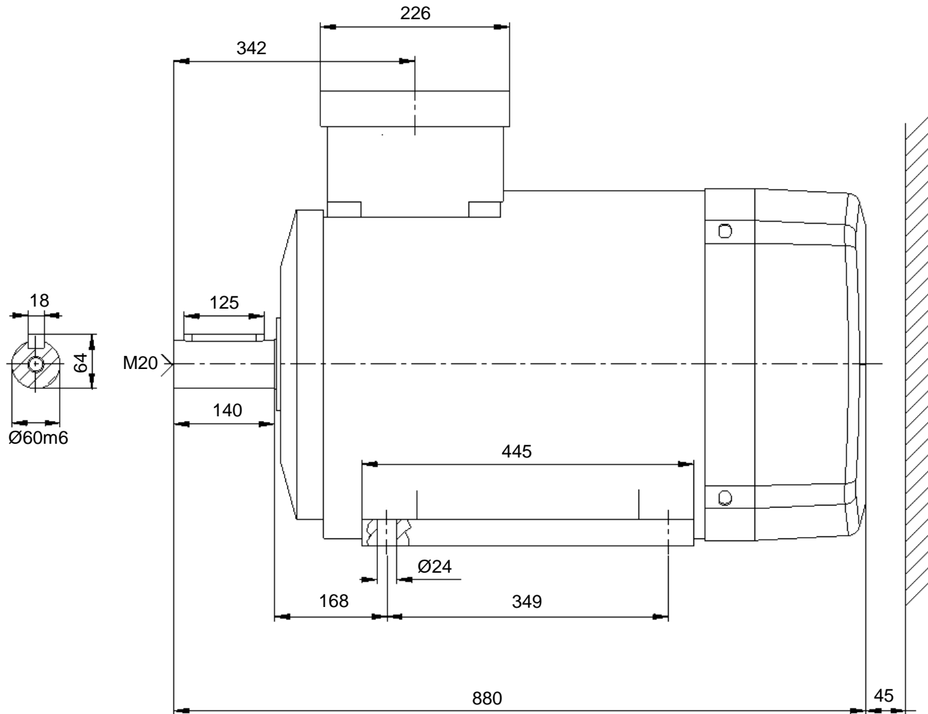
Maßblatt - #715255 - KDG 250 M 2 IE3 ULcsa KT FL NV in Angebot An162717 Position 1 Kabelverschraubung: 2x M63x1,5
